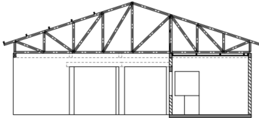
Section D-D
